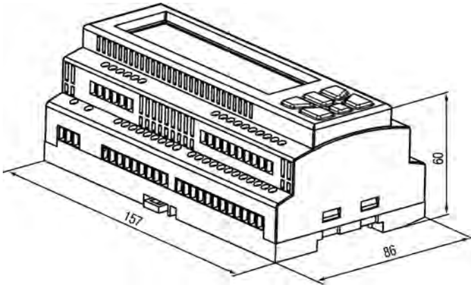
Рисунок А.1 – Габаритный чертеж корпуса для крепления на DIN-рейку 35 мм
