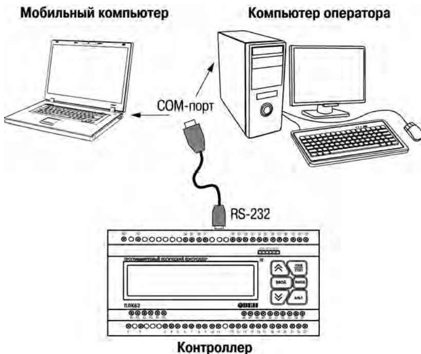
Рисунок 4.1 – Вариант подключения к ПК для программирования контроллера через порт RS-232
