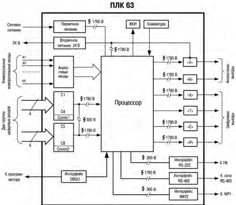
Рисунок 3.2 – Функциональная схема прибора
