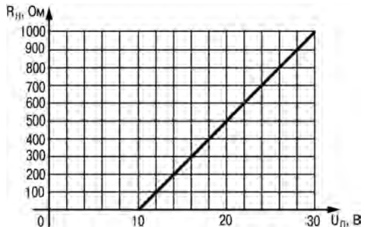
Рисунок 3.4 – График зависимости R_n(U_n)
