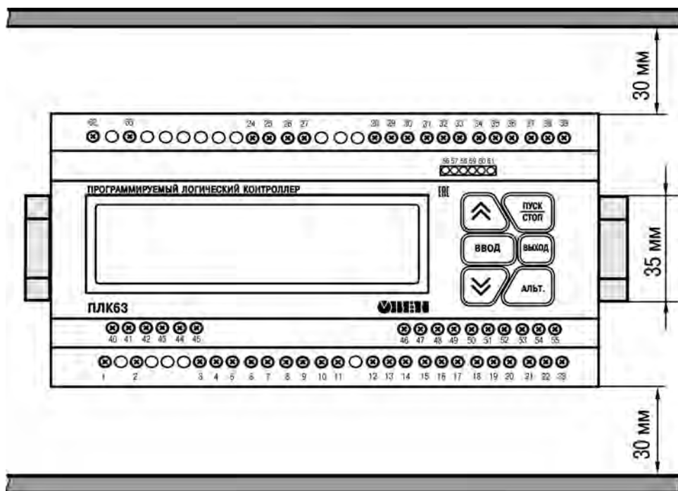
Рисунок А.3 – Расстояние до стенок корпуса ПЛК при монтаже для обеспечения вентиляции
